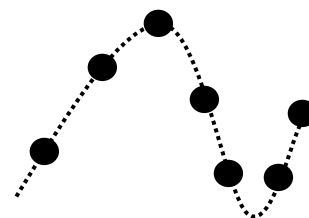
Trajectoire curviligne
