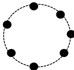
Trajectoire circulaire
