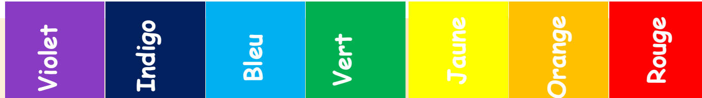
Spectre de la lumière blanche
