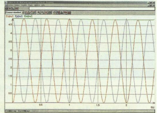
Doc. 9 Représentation des énergies cinétique et potentielle élastique en fonction du temps : quand une énergie est maximale, l'autre est nulle. E_C est représentée en rouge, E_{P_{\text{élas}}} en bleu et E_M en vert.
