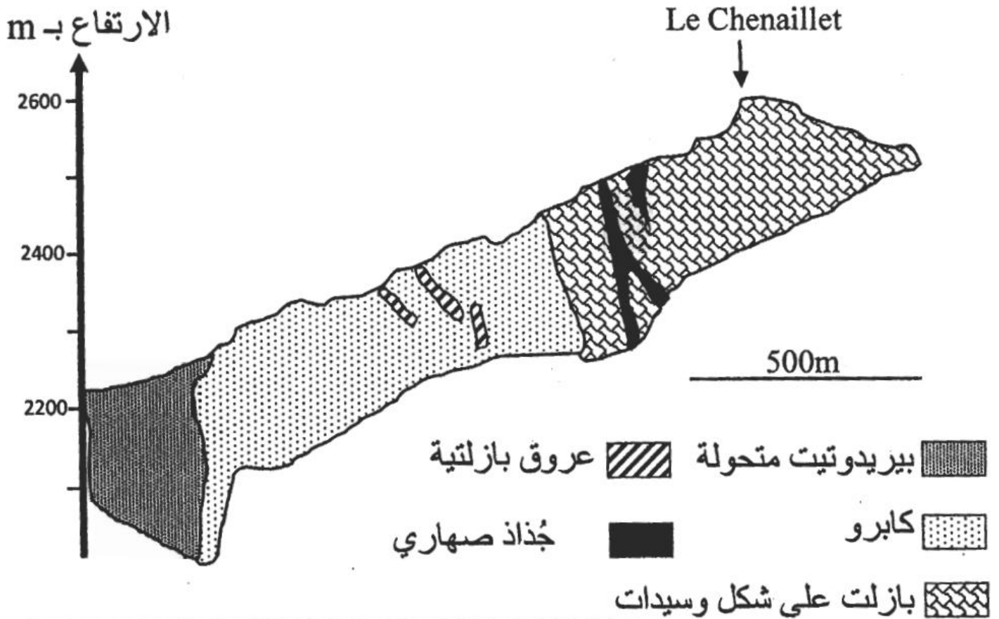
الوثيقة 2: مقطع جيولوجي لأوفيويت كتلة Chenaillet
