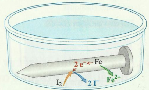
Doc. 13 Le transfert d'électrons entre les réactifs a lieu à la surface du métal.
