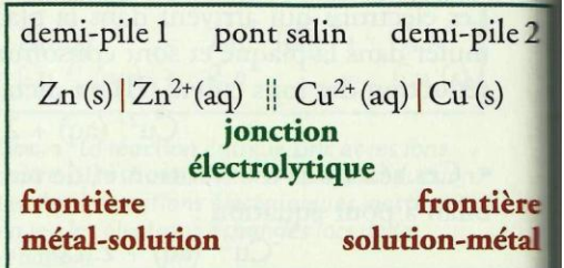
Doc. 7 Schématisation conventionnelle d'une pile.
