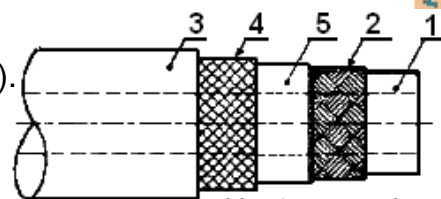
Haute pression
