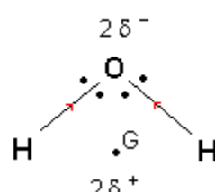
Caractère dipolaire de la molécule d'eau
